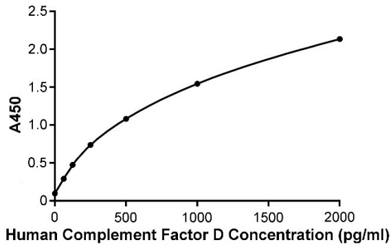
图3. Human Complement Factor D ELISA Kit的标准曲线。实测数据会因实验条件、检测仪器等的不同而存在差异，图中数据仅供参考。
